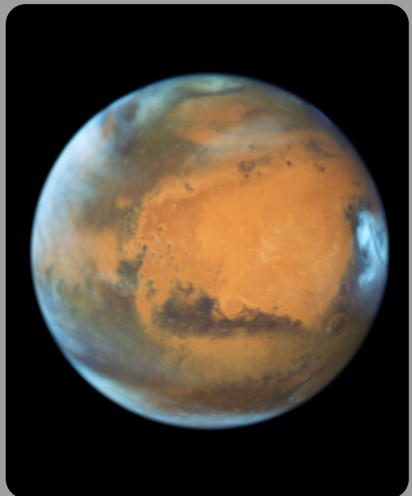
Mars
