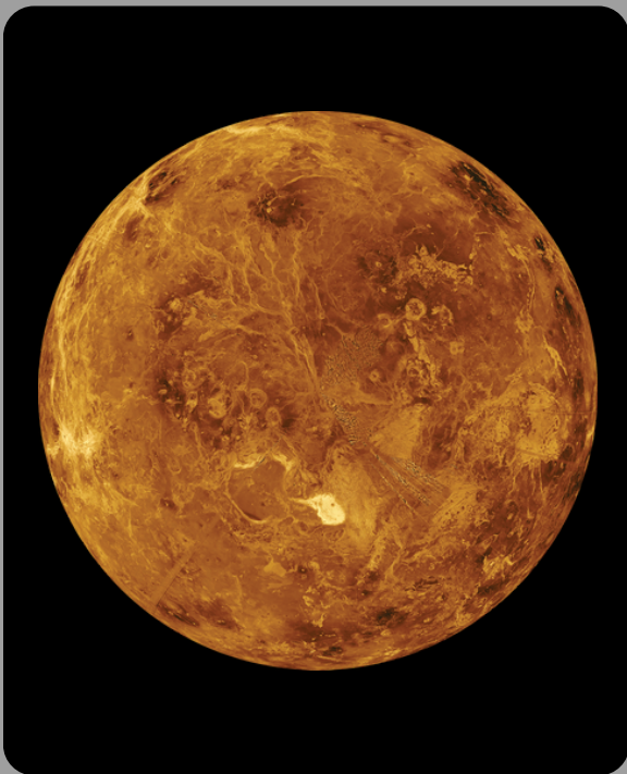
Venus
